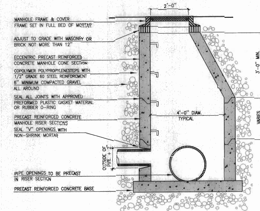
12 Drain Manhole
